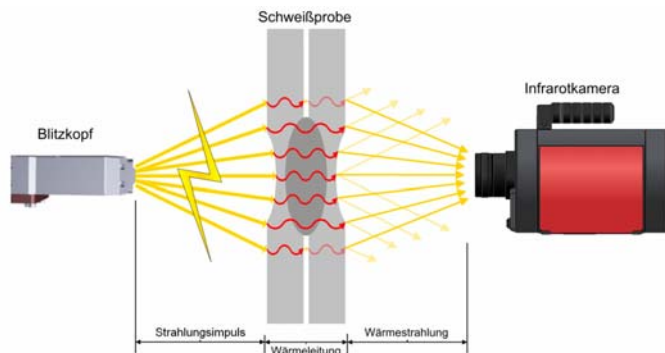
Thermoweld: Vollautomatisches IR-Prüfsystem für Schweißverbindungen im Automobilbau
