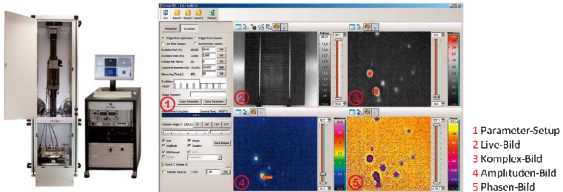
PV-LIT: Automatische Prüfung von Photovoltaik-Zellen
